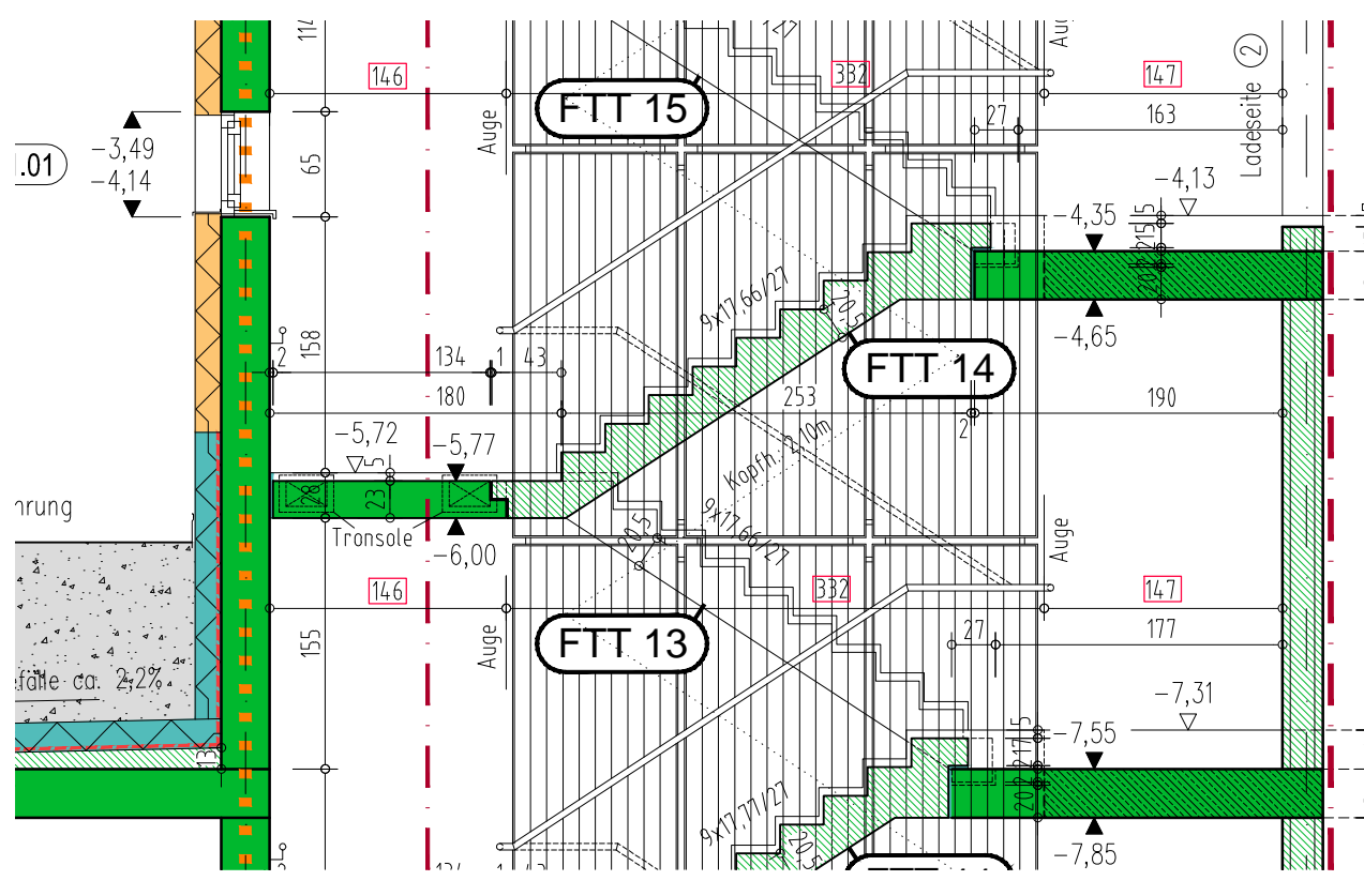
TREPPE FTT 13 I 14 SCHNITT S2 - 1:50
